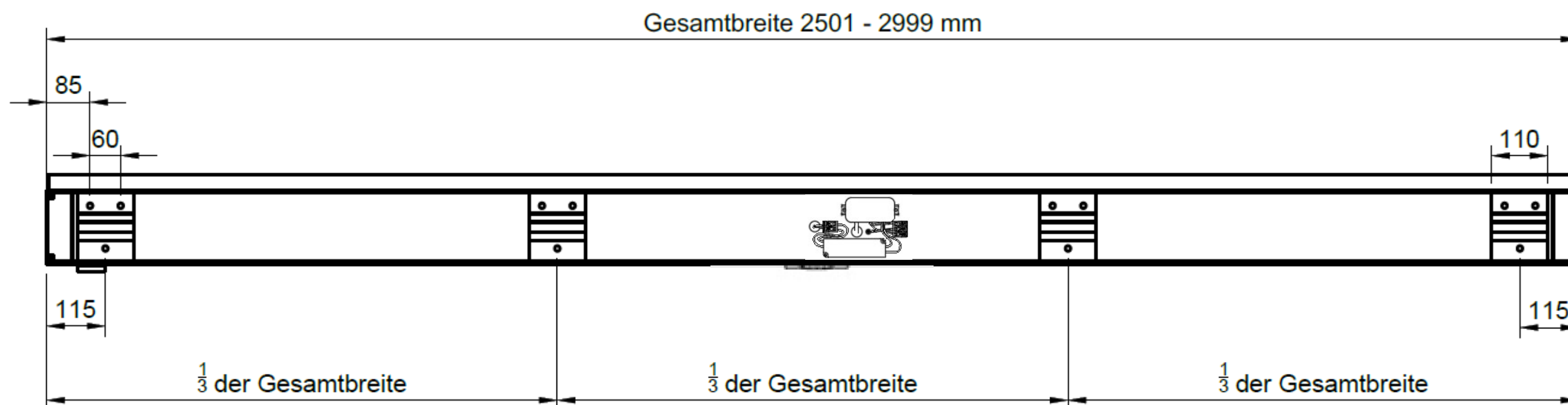
BS Plus 300 Sondermaß 2501 - 2999 mm
