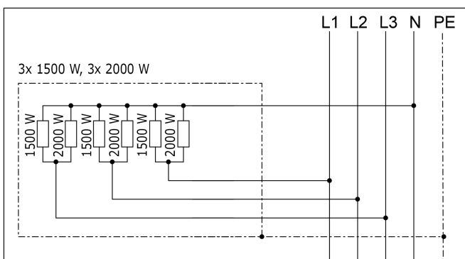
Saunaofen Eterno mit 10,5 kW
