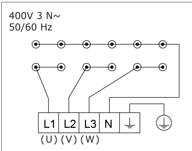
Anschlussplan für Saunaofen Eterno mit 9,0 kW und 10,5 kW
