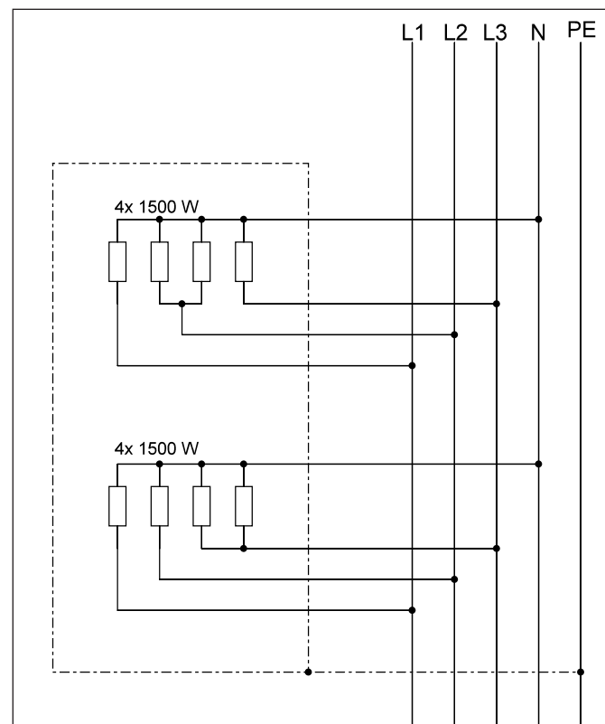
Saunaofen Eterno mit 12,0 kW (2-kreisig)
