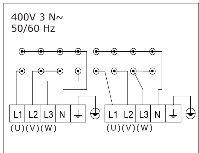
Anschlussplan für Saunaofen Eterno mit 12,0 kW (2-kreisig) mit LSG
