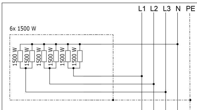
Saunaofen Eterno mit 9,0 kW
